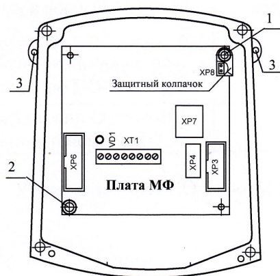
Рисунок 1 - Общий вид преобразователей МастерФлоу
