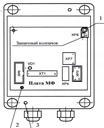
Рисунок 3 - Места пломбирования преобразователей и нанесения знака поверки
